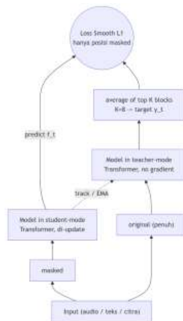
Gambar 3 Arsitektur Data2vec
