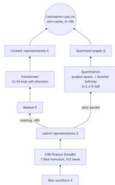
Gambar 2 Arsitektur Wav2vec2 2.0
