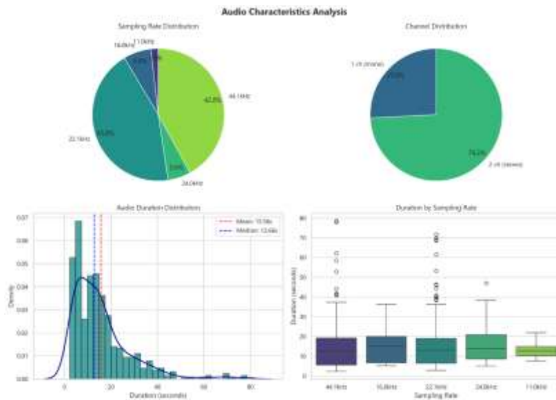
Gambar 5 Karakteristik Audio
